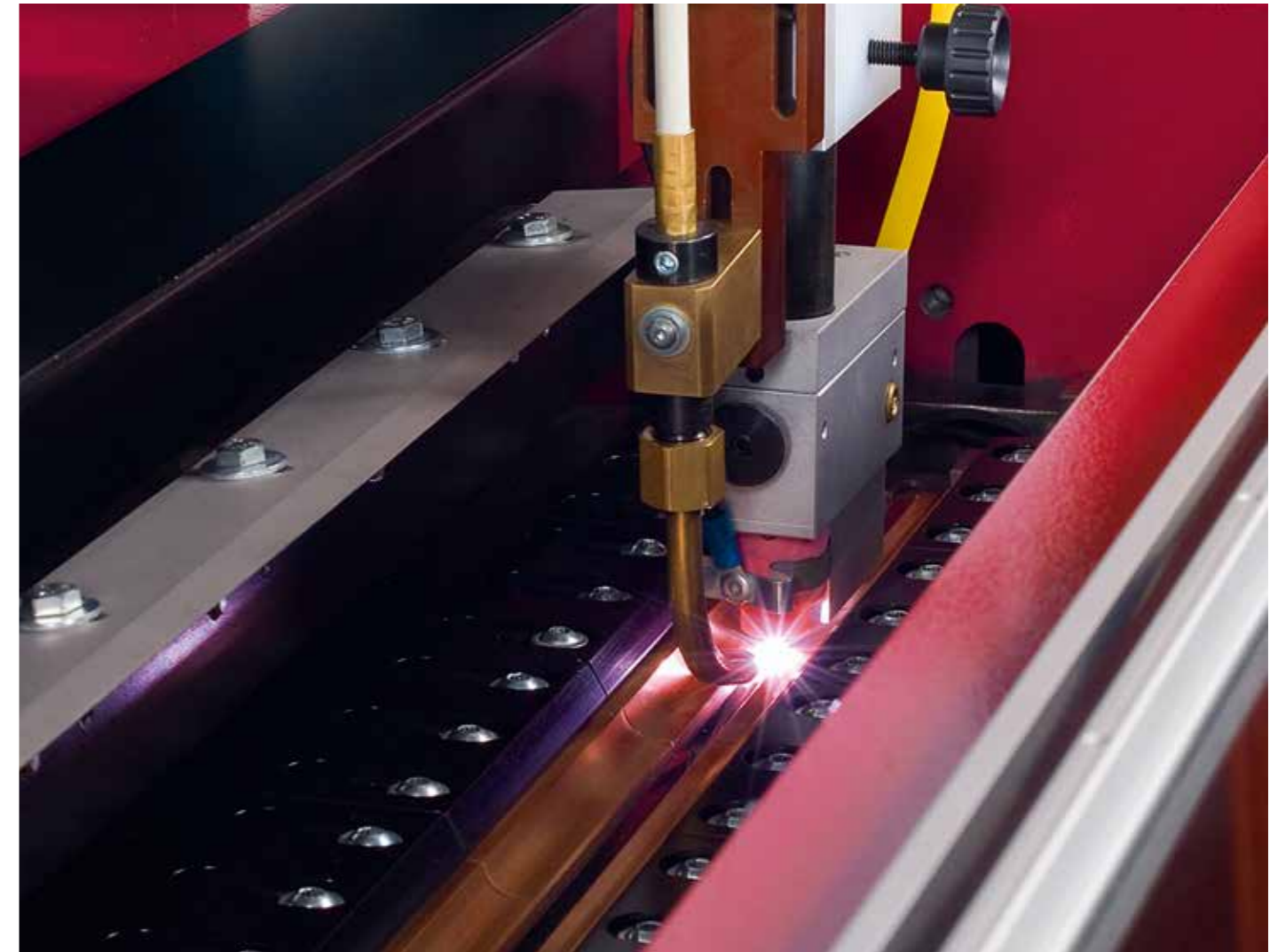
LONGITUDINAL PLASMA WELDING
